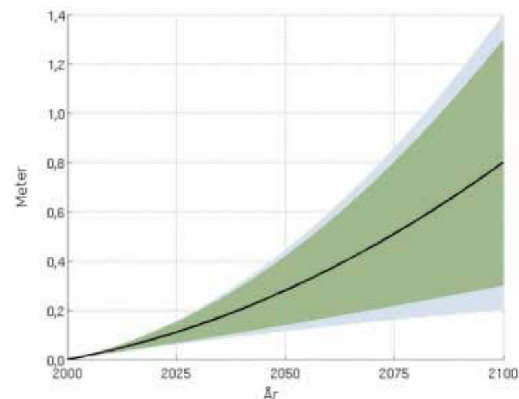
DMI's bedste bud på havvandstandstigninger mellem år 2000-2100, når der ses bort fra landhævning. Den sorte kurve viser middelværdien, mens det grønne og blå areal viser usikkerheden hhv. globalt og omkring Danmark.
