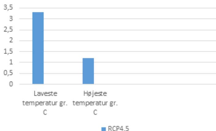
ÆNDRING I TEMPERATURER ÅR 2070
