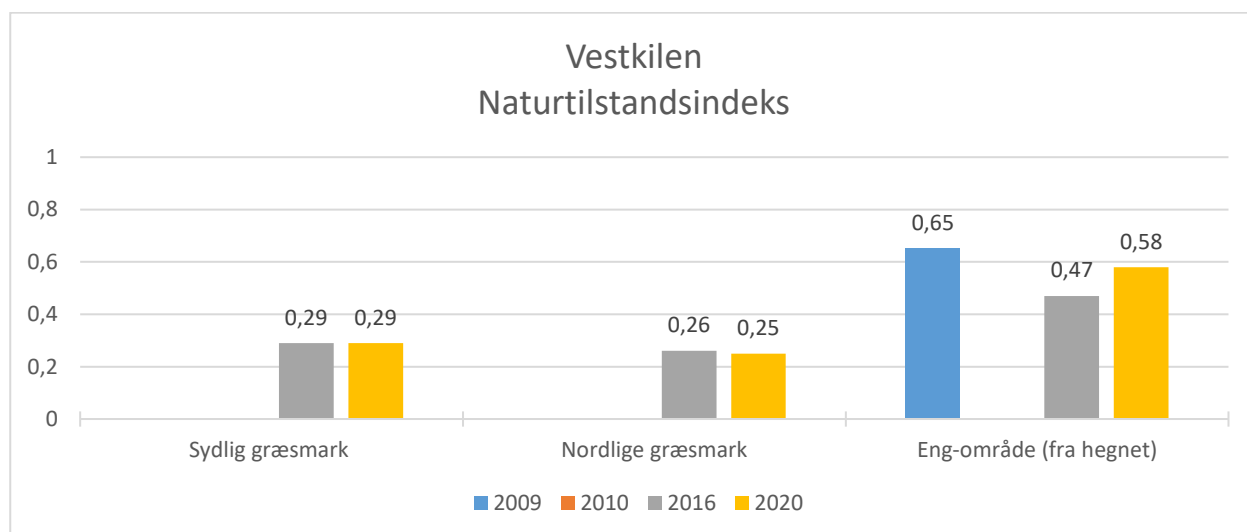
Figur 49: Vestkilen – Naturtilstandsindex.
