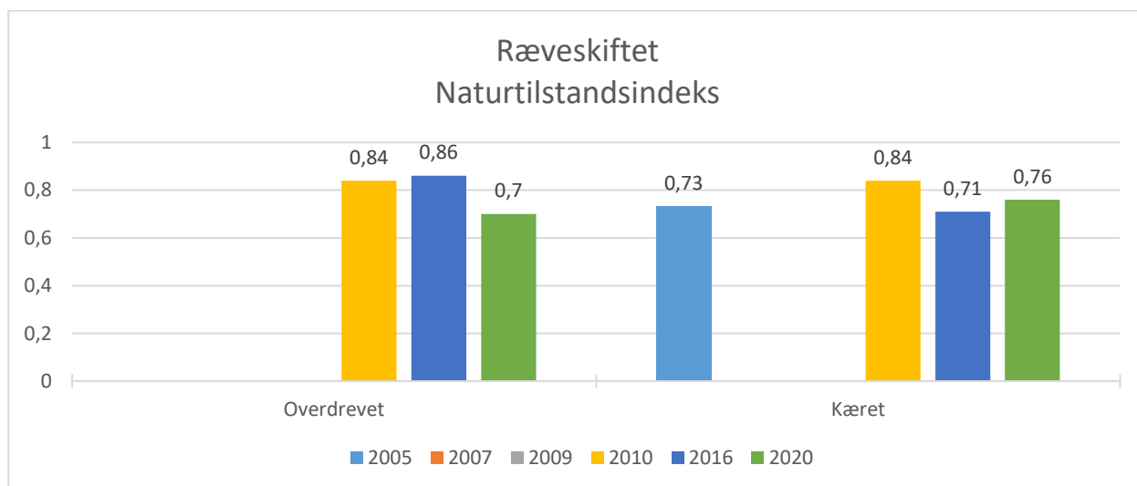
Figur 51: Ræveskiftet – Naturtilstandsindex.
