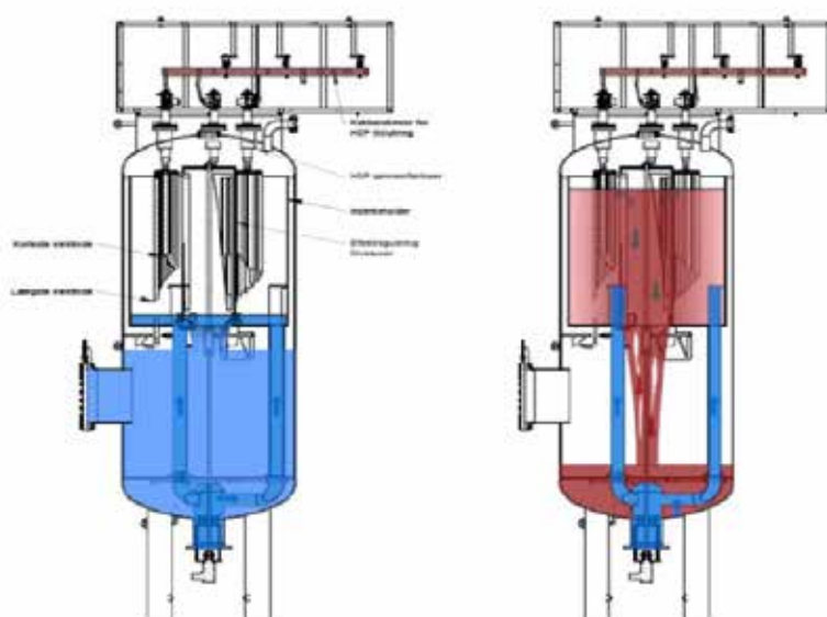
FIGUR 16: SNIT I EL-KEDEL, DER ILLUSTRERER EFFEKTRÉGULERINGEN MED VARIATION AF VÆSKETANDEN OMKRING ELEKTRODERNE
